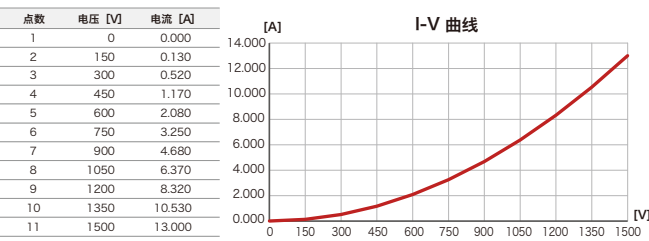
PXZ20K-1500 CC模式的设定例
