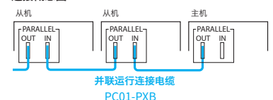
连接概念图
